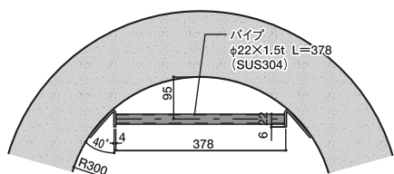
支持金物図
